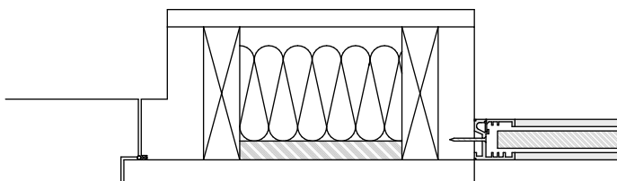
Alt 3: Profil i front Aluprofil monterad i front på portal
